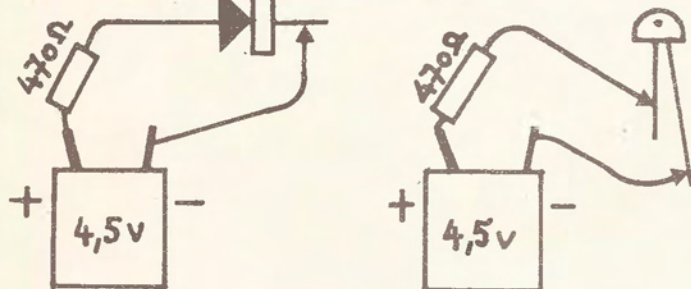
Câblage d'une nappe sur les diodes.
