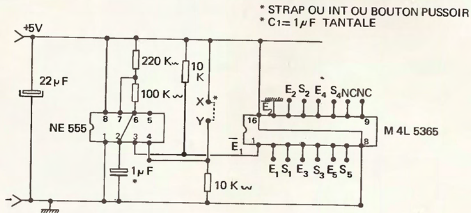
Montage final de la carte répétition caractères.
