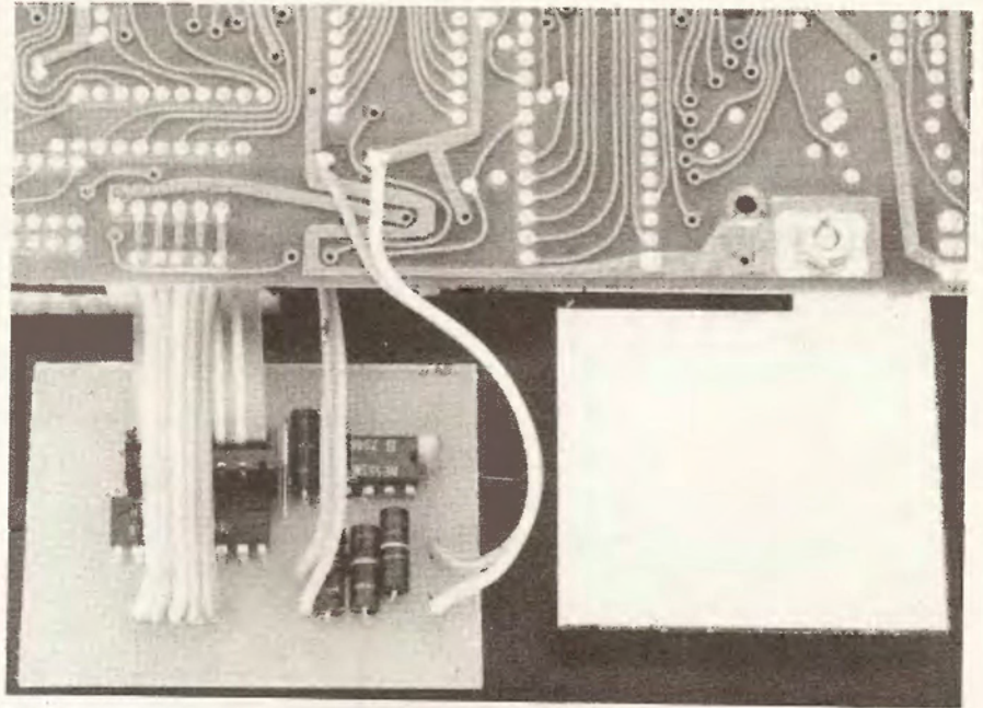
Montage final de la carte répétition caractères.
