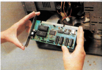
Manuseie as placas com cuidado, sem tocar nos chips
