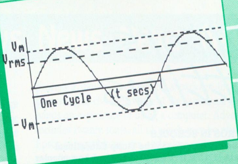
AC Circuits
