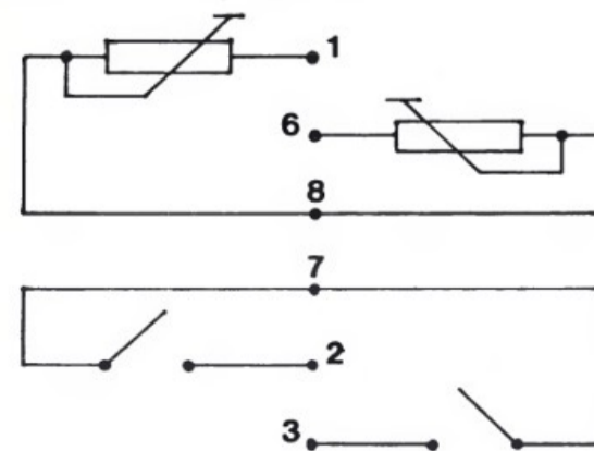
Rys. 2. Schemat elektryczny zespołu wioselek.
