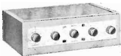
▲ Fig. 11 - Amplificatore integrato 30 watt, HF-32.
