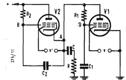
Fig. 3 ► Circuito che impiega, allo scopo di avere una certa potenza, due pentodi. La soluzione per l'alimentazione delle griglie schermo, qui presentata ha l'inconveniente di avere la resistenza di griglia schermo in parallelo (dal punto di vista della componente alternata) con il carico.
