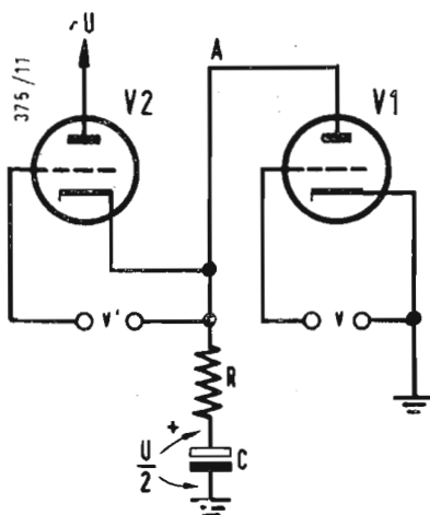
Fig. 3 ► Circuito che impiega, allo scopo di avere una certa potenza, due pentodi. La soluzione per l'alimentazione delle griglie schermo, qui presentata ha l'inconveniente di avere la resistenza di griglia schermo in parallelo (dal punto di vista della componente alternata) con il carico.
