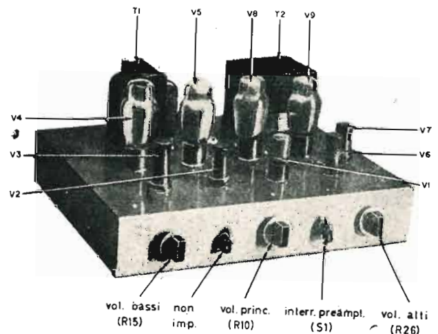
▲ Fig. 1 bis - Disposizione delle valvole e dei controlli. Il canale dei bassi è a sinistra e quello degli alti a destra.
