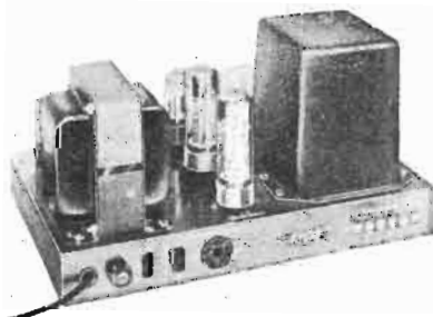
▲ Fig. 13 - Amplificatore di potenza 35 watt, HF-35.
