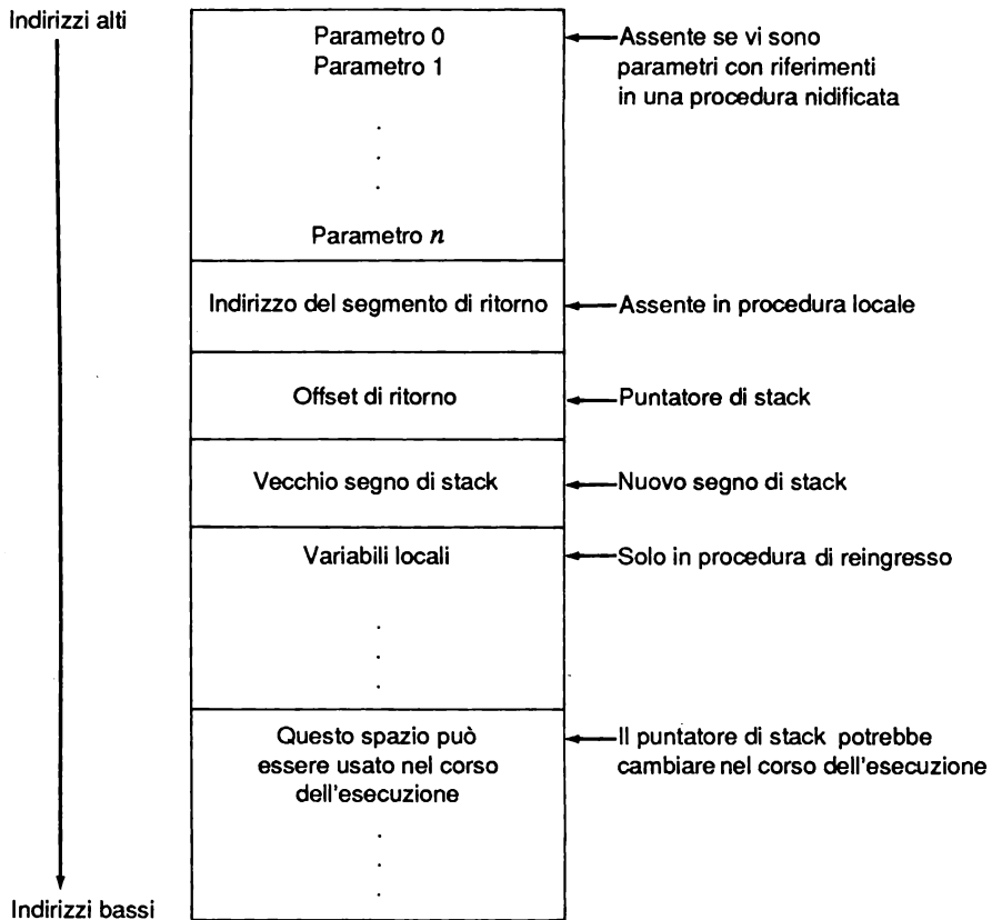
Figura D.2 Aspetto dello stack durante l'esecuzione di un'istruzione CALL
