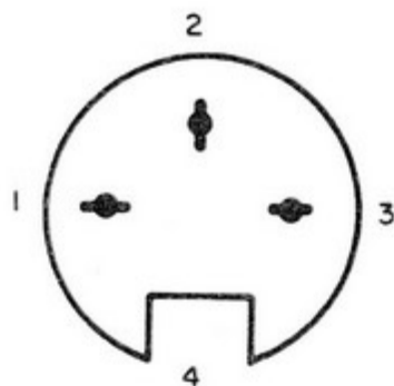
Pinagem do conector de vídeo
