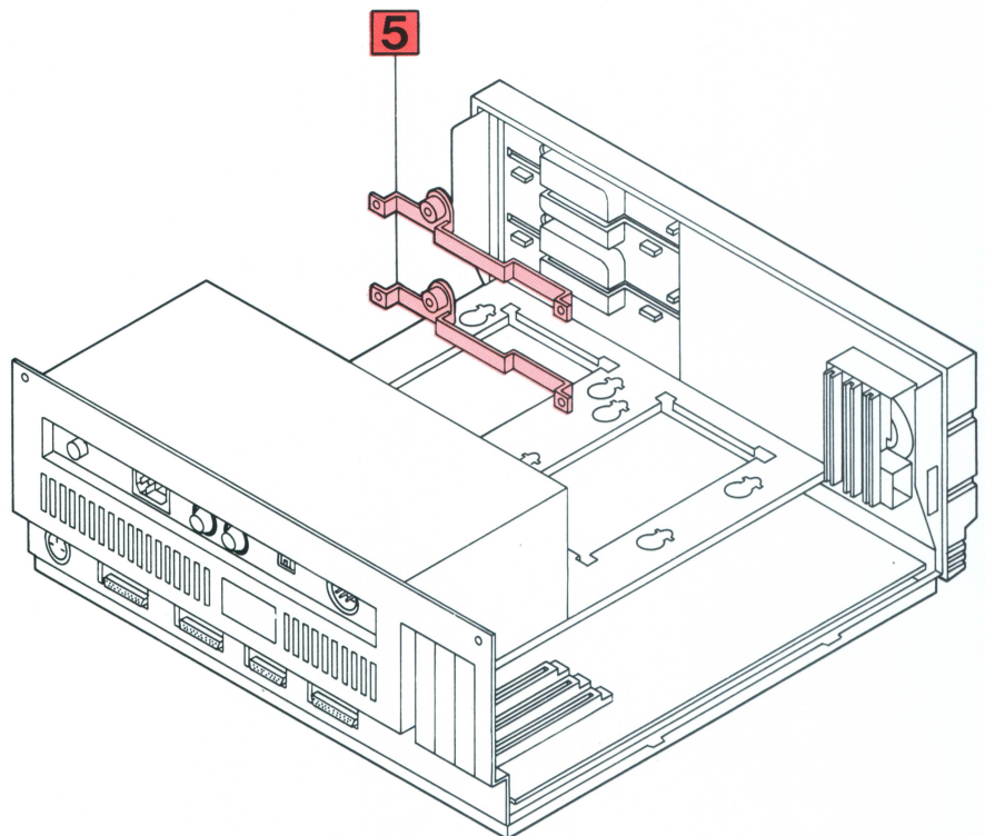
5. Painel de fechamento Quando a instalação for de apenas um disco, retire somente o painel de fechamento da fenda "A"
