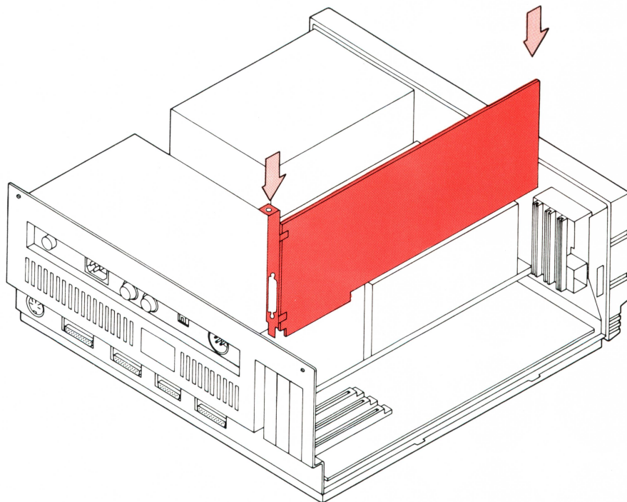
Colocação correta da placa de expansão
