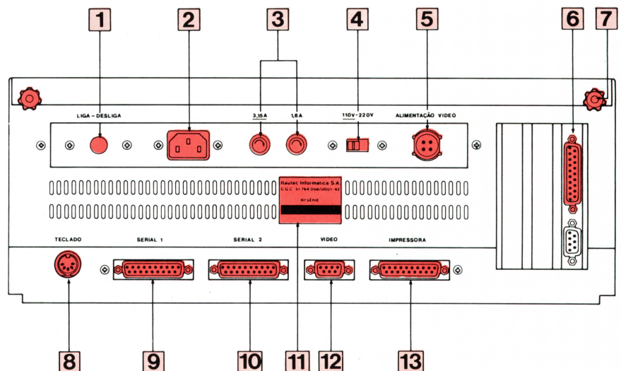
Localização dos conectores do painel traseiro do módulo básico
