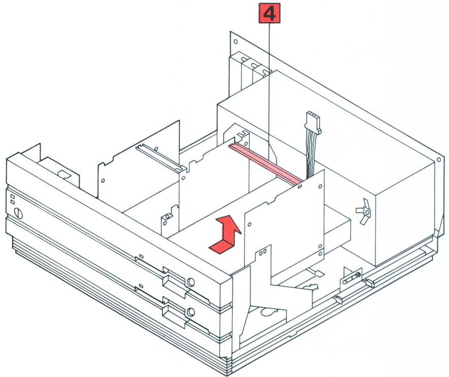
4. Alça para facilitar a movimentação do conjunto
