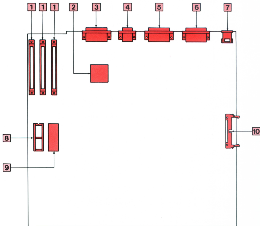
Lay-Out da Placa Básica do IS 30 plus II
