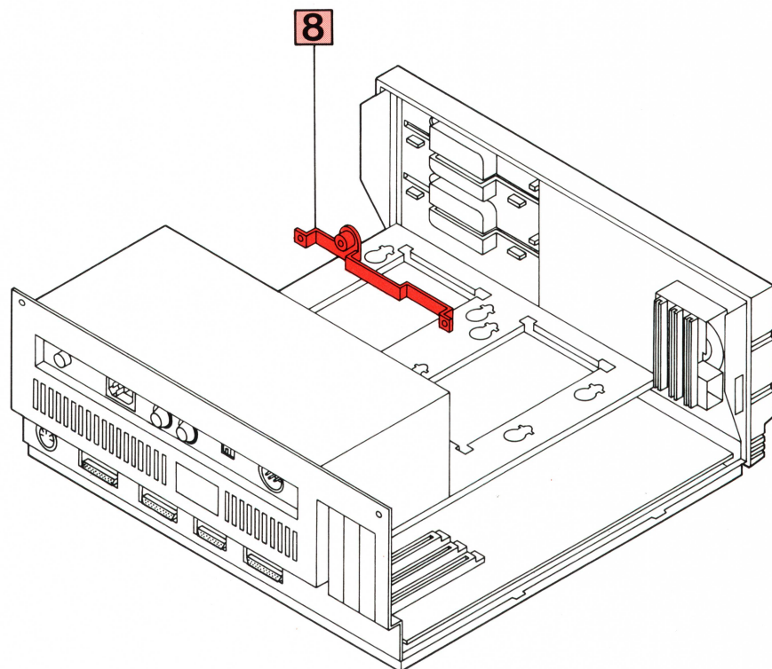
8. Painel de fechamento da "fenda" B
