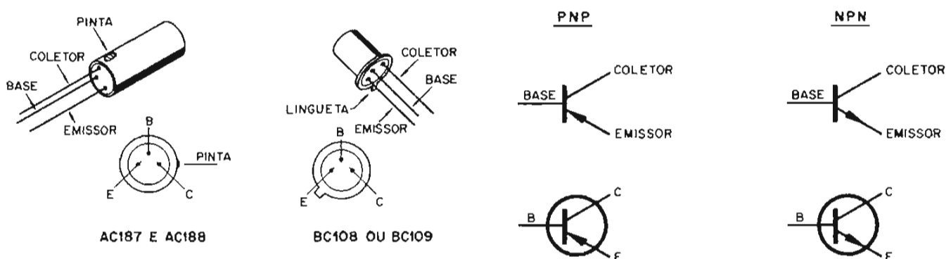
Figura 7 - Identificação dos transistores e disposição dos terminais.
