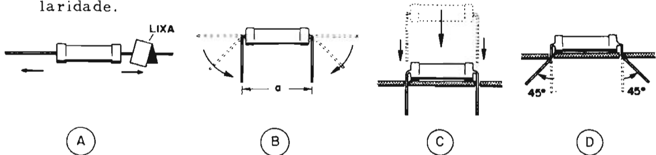
Figura 5 - Preparação, montagem e fixação mecânica de componente numa placa de fiação impressa.
