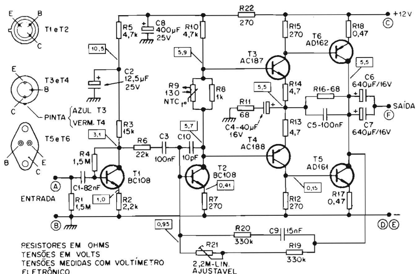
Figura 20 - Circuito esquemático do módulo amplificador M-110 com modificações para operar em 12V.
