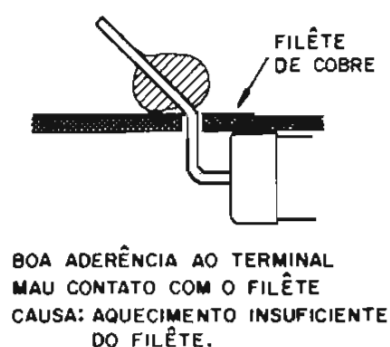
Figura 3 - Defeitos mais comuns e execução correta de soldagens.
