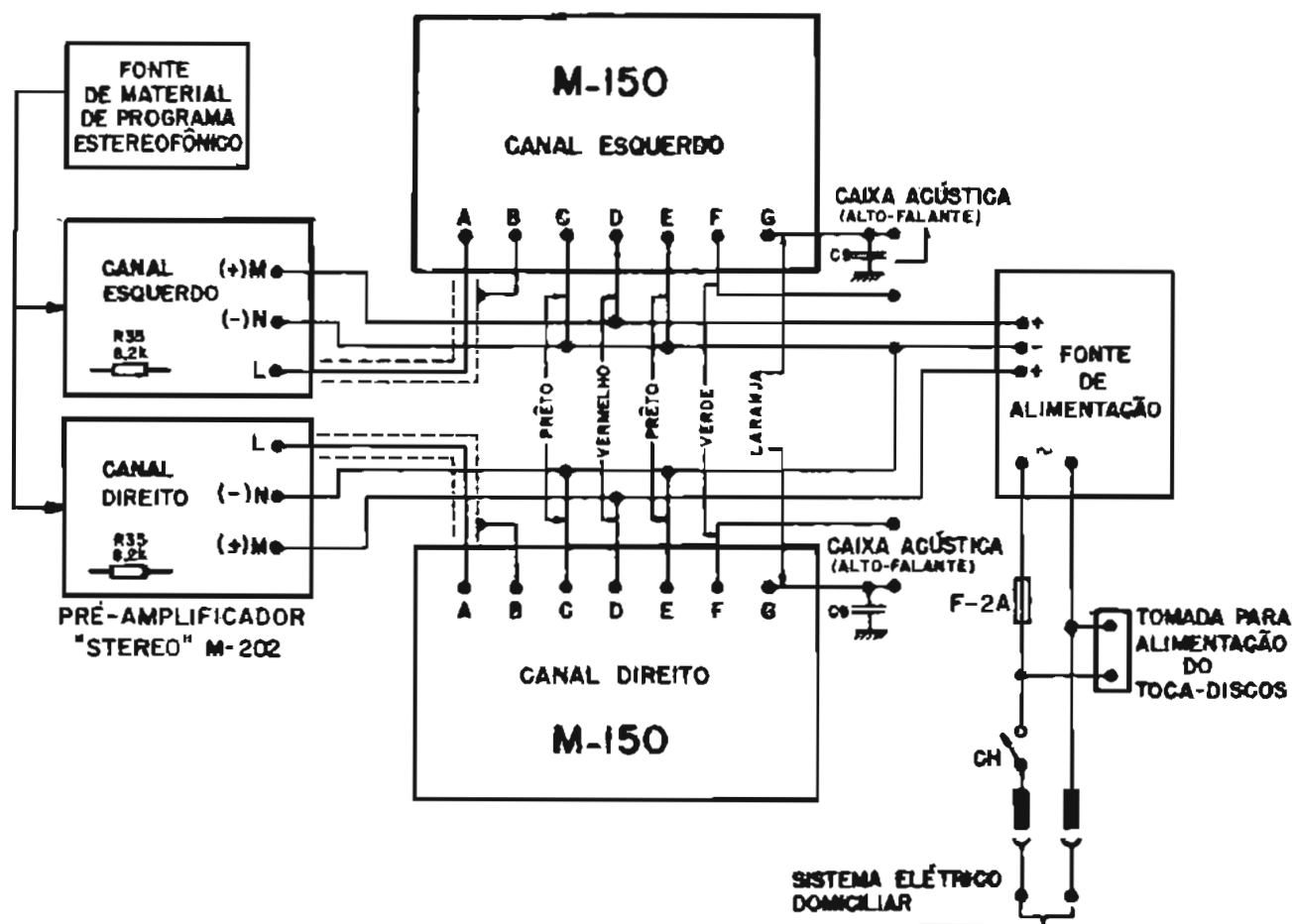
Figura 1-1 - Interligações num aparelho estereofônico.
