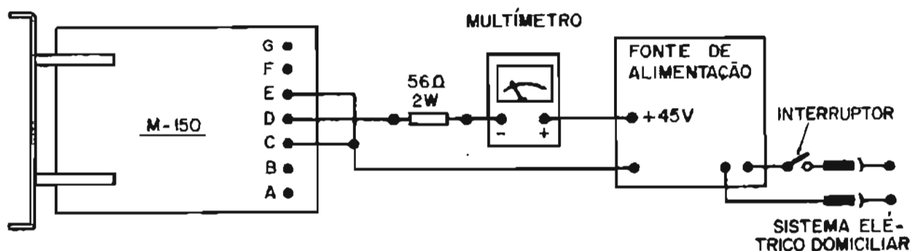
Figura 12 - Teste de funcionamento do módulo M-150.
