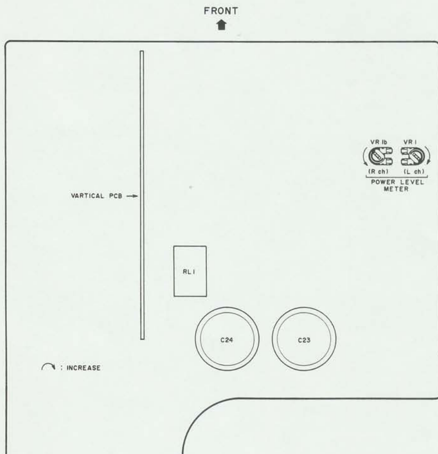
Fig. 6-2 Main-Amp PCB
