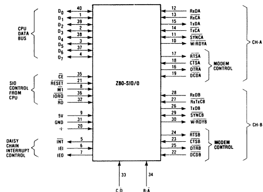
FIG. 9 -- Z80-SIO/0 PIN CONFIGURATION
