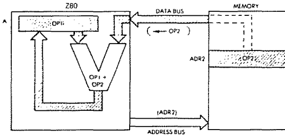
Fig. 3.3: ADD A, (HL)
