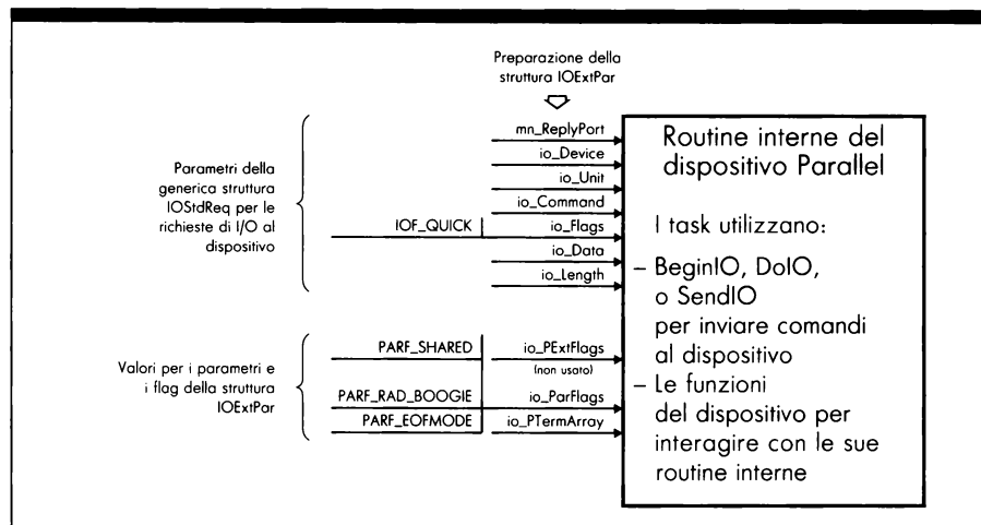
Figura 5.2a: Gestione delle funzioni e dei comandi previsti dal dispositivo Parallel (input)
