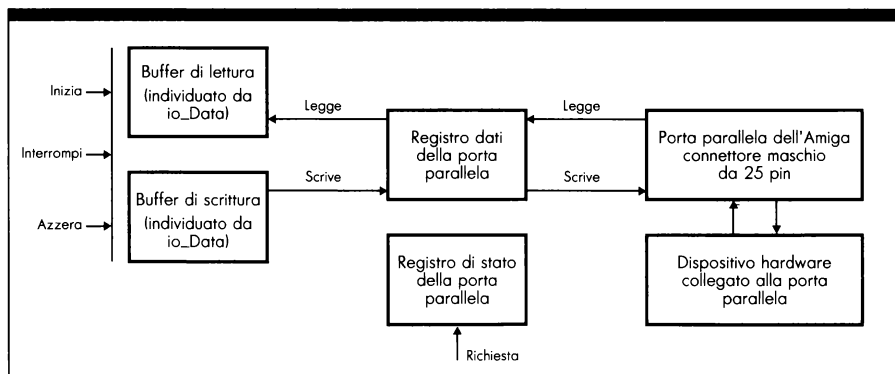
Figura 5.1: Operazioni di lettura e scrittura del dispositivo Parallel
