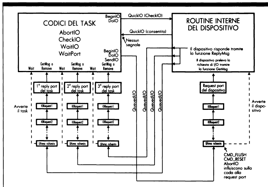
Figura 1.2: Interazioni fra task e dispositivo quando il task dispone di tre reply port
