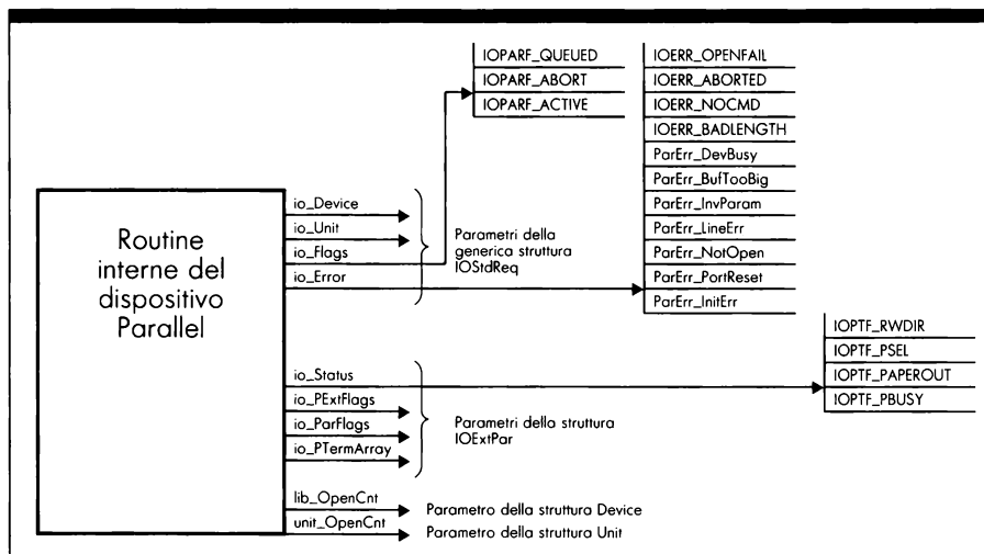
Figura 5.2b: Gestione delle funzioni e dei comandi previsti dal dispositivo Parallel (output)
