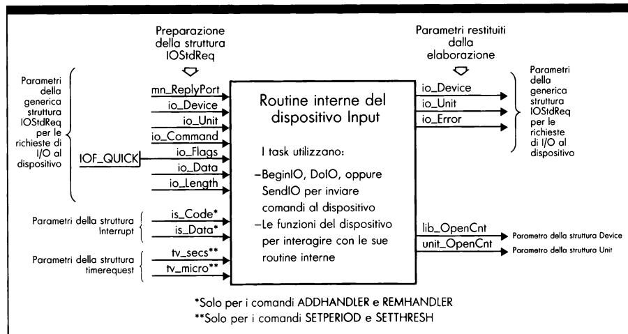
Figura 7.2: Gestione delle funzioni e dei comandi previsti dal dispositivo Input
