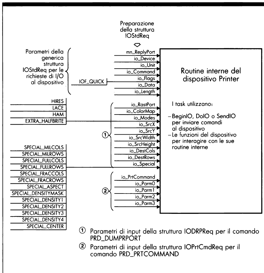
Figura 11.2a: Gestione delle funzioni e dei comandi previsti dal dispositivo Printer (input)
