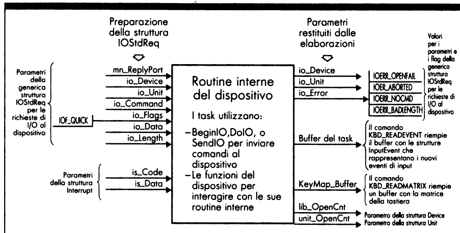
Figura 9.3: Gestione delle funzioni e dei comandi previsti dal dispositivo Keyboard
