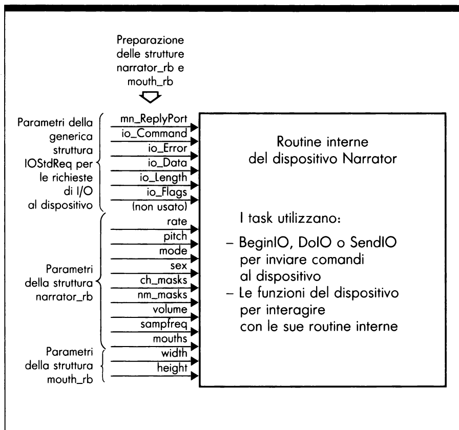
Figura 4.2a: Gestione delle funzioni e dei comandi previsti dal dispositivo Narrator (input)
