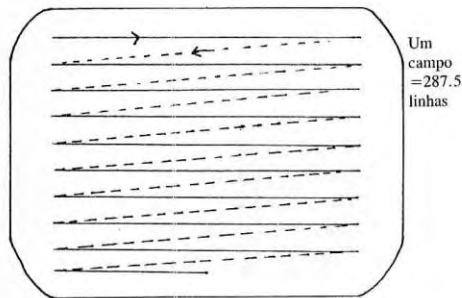
Face do tubo catódico
