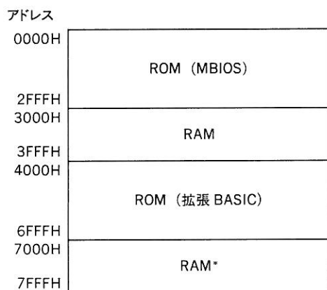
図 7.28 バンク 0 (MBIOS、拡張 BASIC 動作時)
