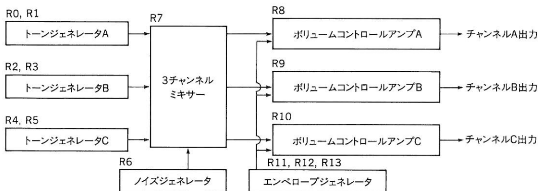
図 6.1 PSG のブロックダイアグラム
