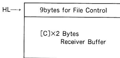
図 7.7 FCB の形式
