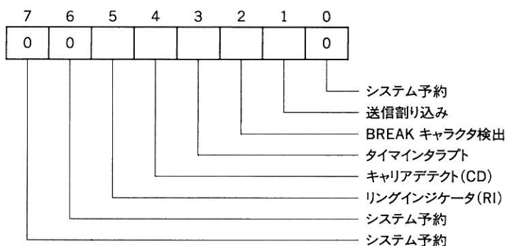
図 7.5 DVINFB の形式
