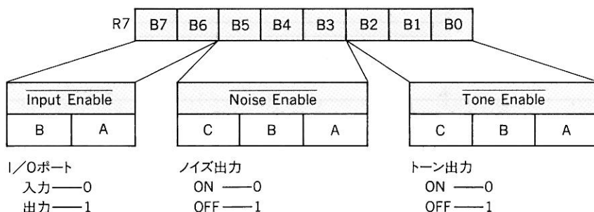
図 6.5 各チャンネルの出力選択
