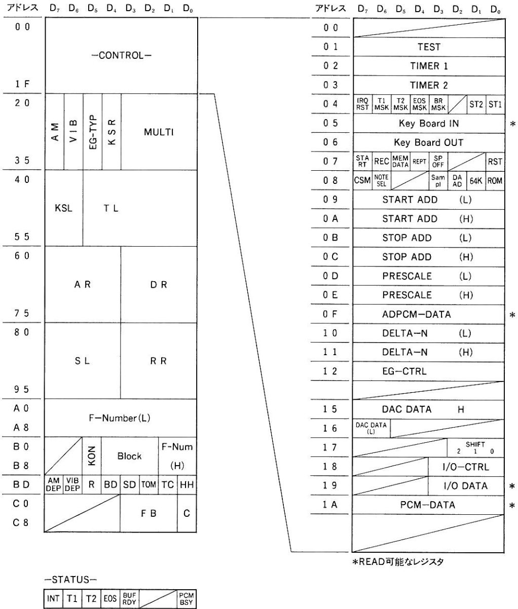
図 7.39 MSX-AUDIO のレジスタマップ
