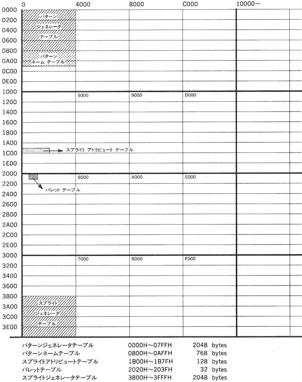
図 A.5 SCREEN 3 VRAM マップ
