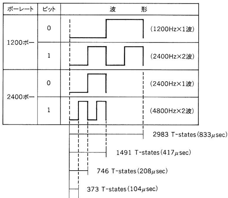
図 6.10 1ビットの構成
