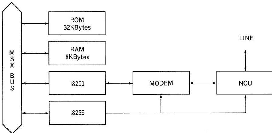
図 7.8 MSX MODEM の基本構成
