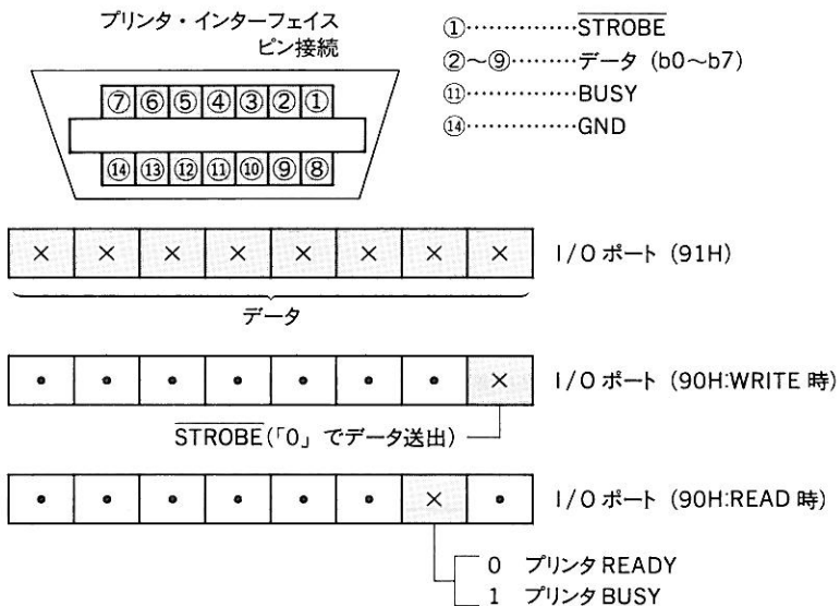
図 6.18 プリンタインターフェイス
