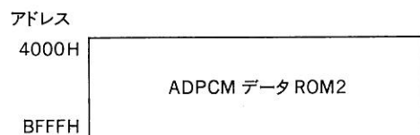
図 7.31 バンク 3 (ADPCM データ ROM2 読み出し時)
