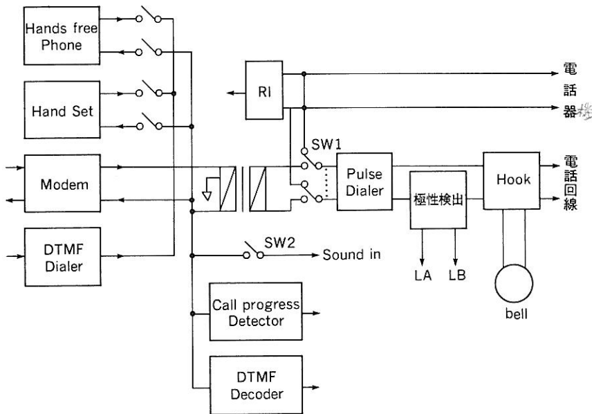
図 7.9 NCUの構成
