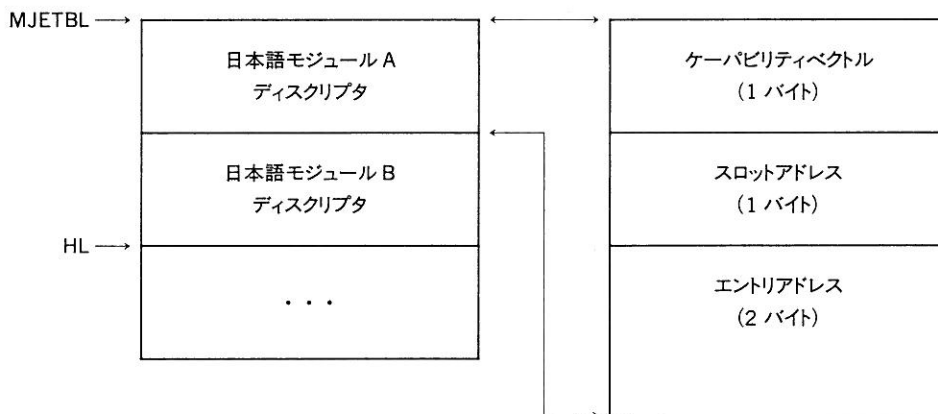
図 7.48 RETURN 情報の形式
