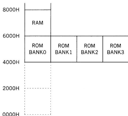
図 7.10 メモリの構成
