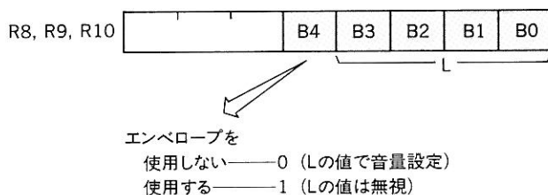
図 6.6 音量の設定
