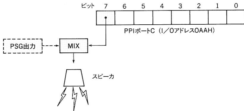
図 6.9 1ビットサウンドポート
