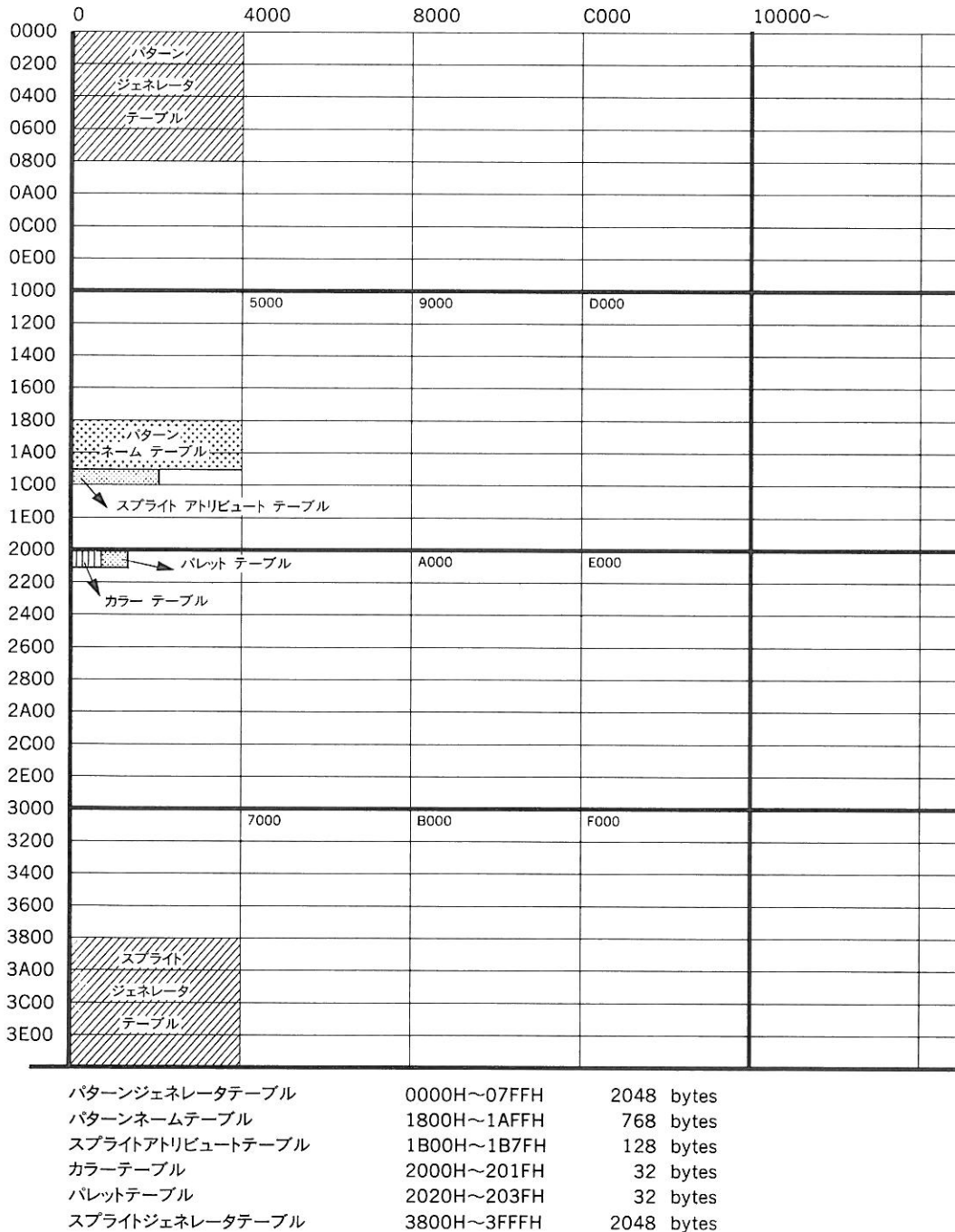
図 A.3 SCREEN 1 VRAM マップ
