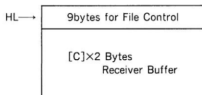
図 7.16 FCBの形式
