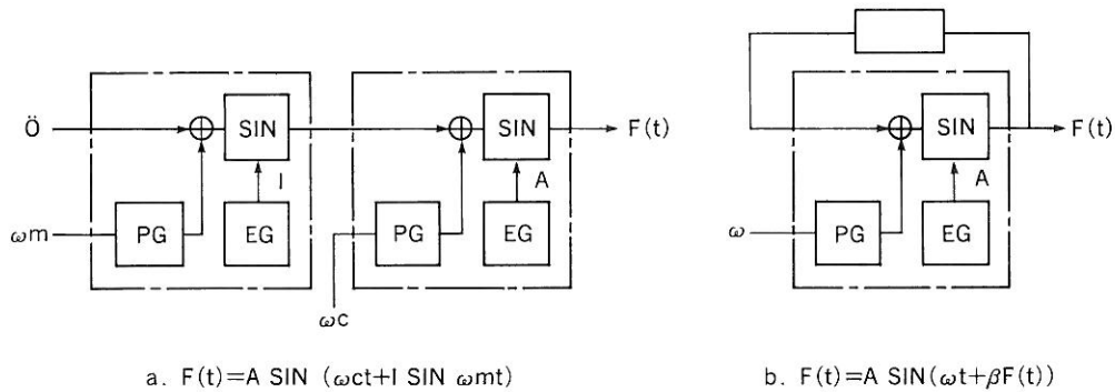
図 7.23 ユニットセルによる FM 方式の表現
