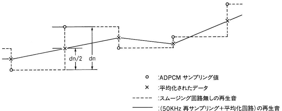
図 7.38 ADPCM 音声合成波形
