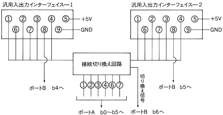
図 6.19 汎用入出力インターフェイス
