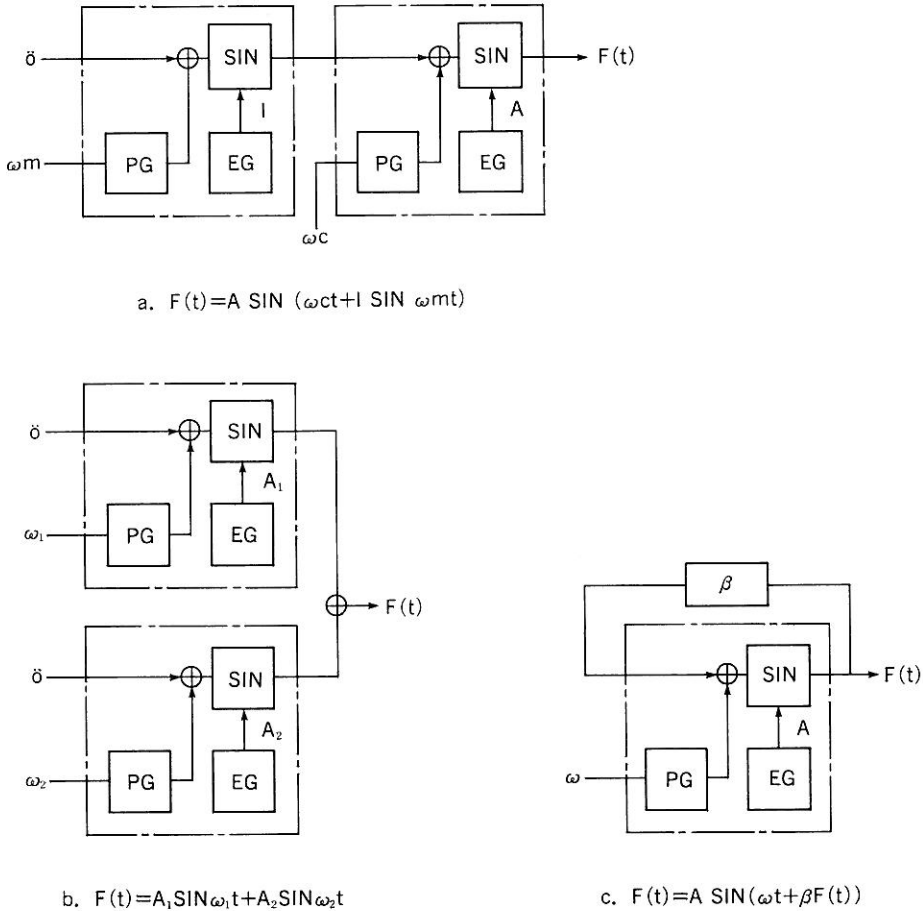
図7.37 ユニットセルによるFM方式の表現
