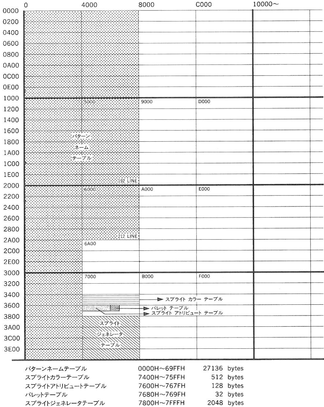
図 A.7 SCREEN 5, 6 VRAM マップ
