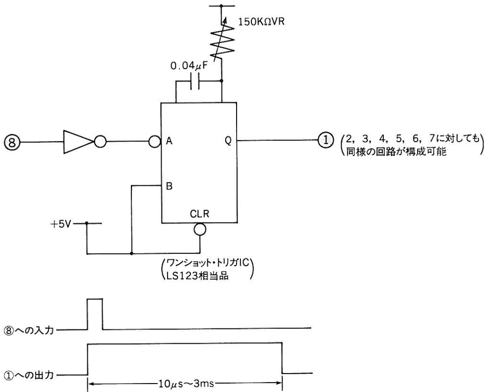
図 6.22 パドル回路図
