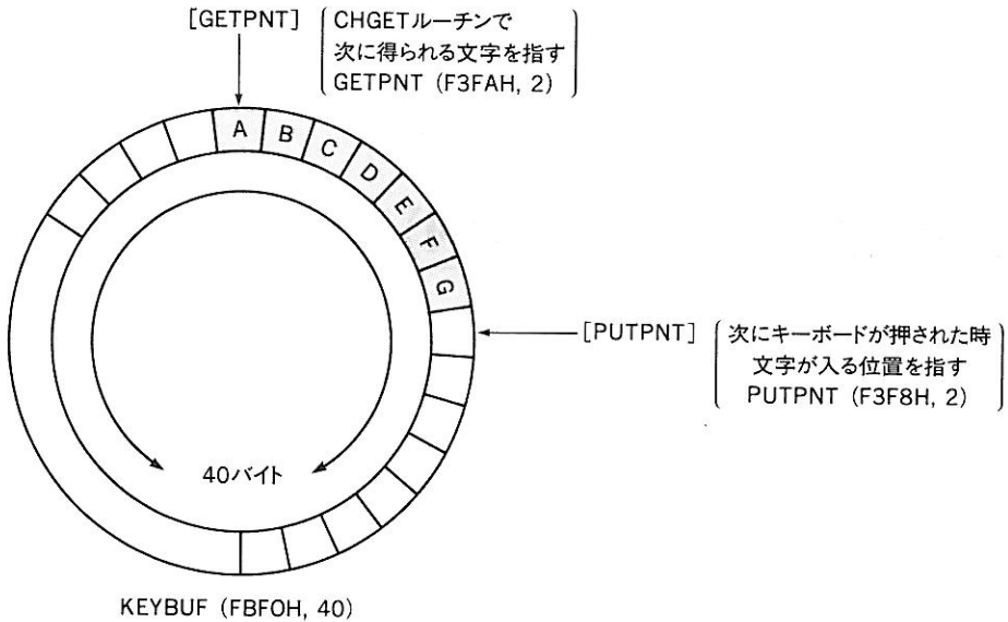
図 6.16 リング状のキーボードバッファ
