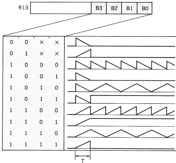
図 6.8 エンベロープの波形の設定
