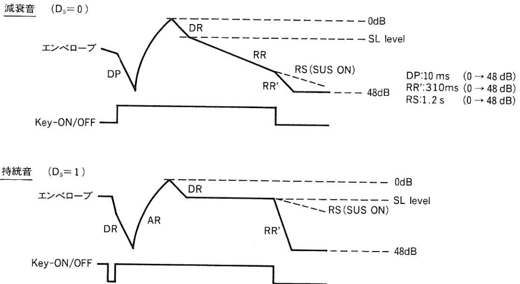
図 7.26 OPLL の減衰音、持続音のエンベロープ
