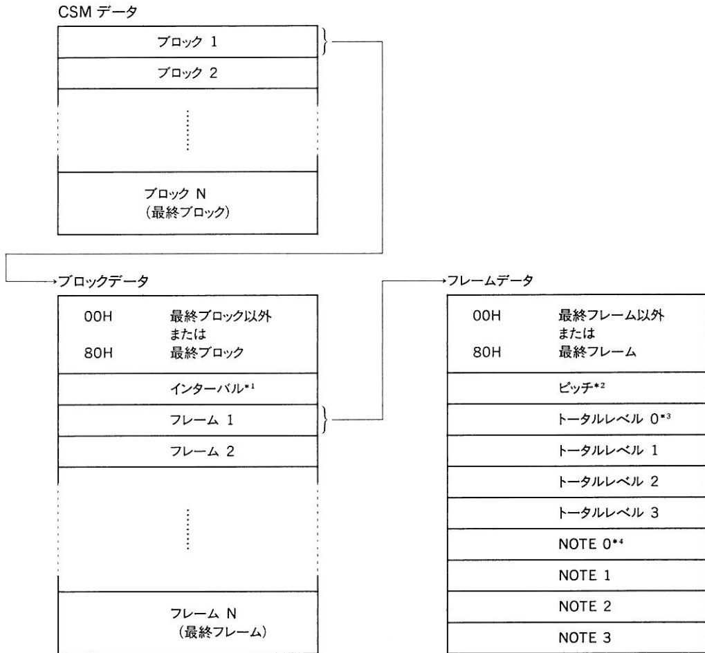
図 7.36 CSM データの形式
