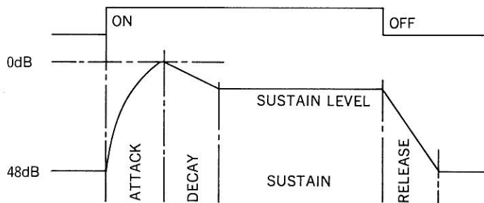
図 7.42 エンベロープ波形
