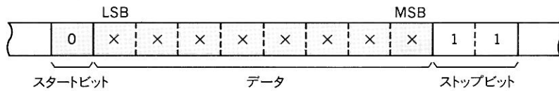
図 6.11 1 バイトの構成
