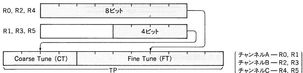
図 6.3 音程の設定
