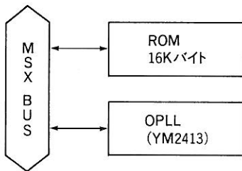
図8.18 MSX-MUSICのメモリ構成
