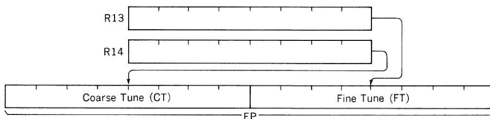
図 6.7 エンベロープ周波数の設定
