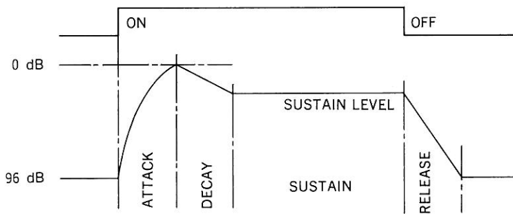
図 7.27 OPLL のエンベロープ波形
