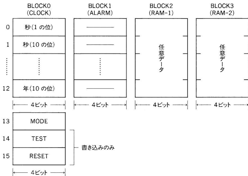
図 6.23 CLOCK-IC の構造
