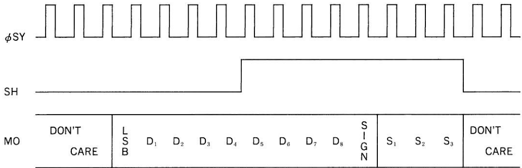
図 7.43 出力タイミング
