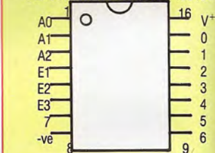
DECODIFICADOR DE 3 A 8 74LS138
