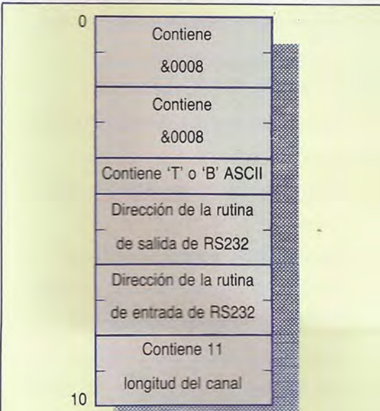
Estructura del canal del RS232
