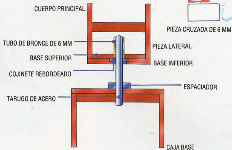
ELEVACION LATERAL
