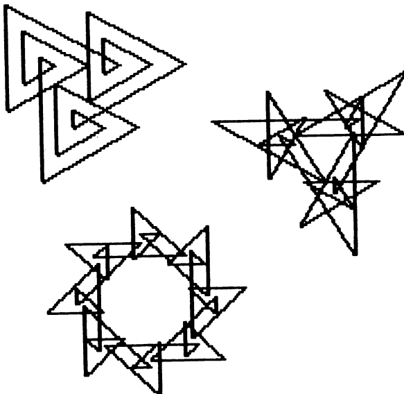
Figura 8.23 Altre spiraloïdi
