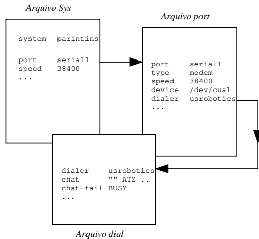
Figura 12.1: Interação dos Arquivos de Configuração do Taylor UUCP
