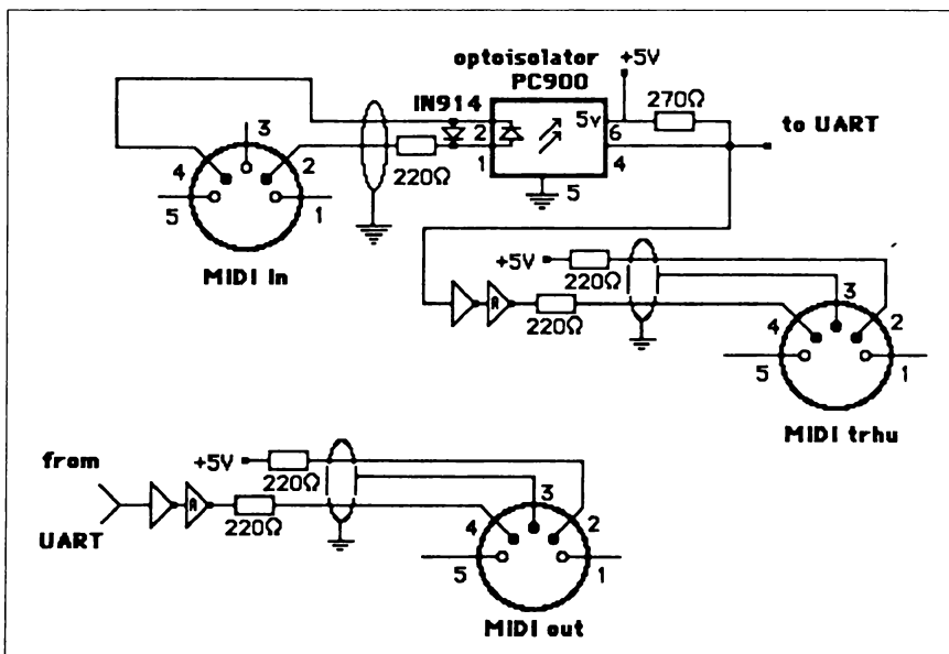
Fig. 2.1 I connettori MIDI.
