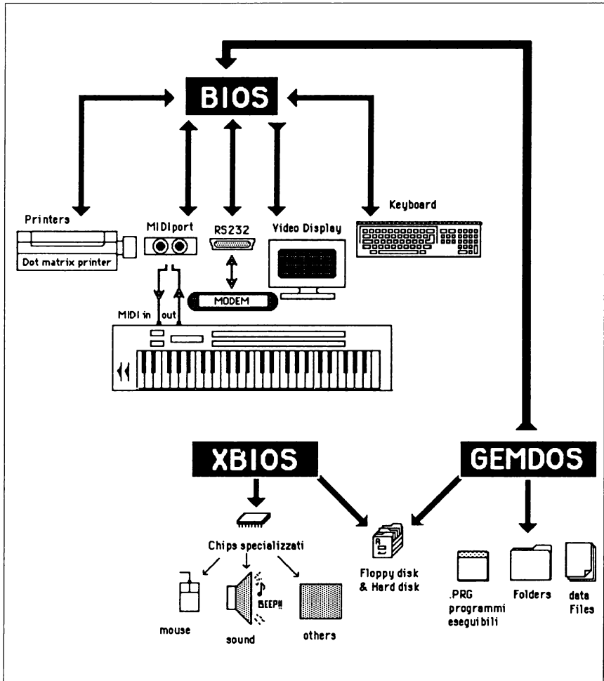
Fig. 4.1 Il TOS™ (The Operating System) dell'Atari e la sua struttura modulare.
