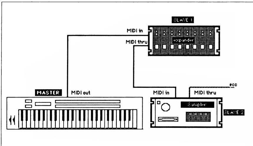
Fig. 2.2 Una architettura MIDI in parallelo.
