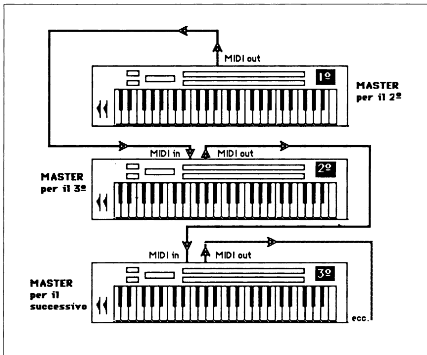
Fig. 2.3 Architettura MIDI in serie.
