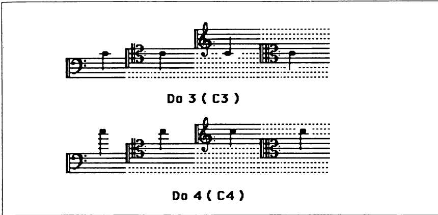
Fig. 1.8 Equivalenza tra scritte della stessa nota in chiavi diverse.
