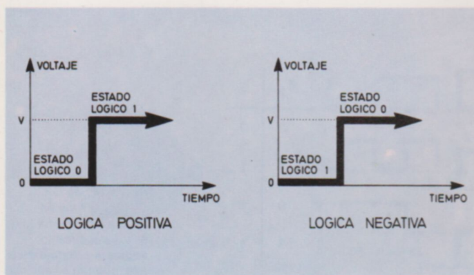
En lógica positiva se asigna el estado lógico «1» al nivel de tensión más alto. Por el contrario, en lógica negativa, el «1» lógico se corresponde con el nivel de tensión inferior.
