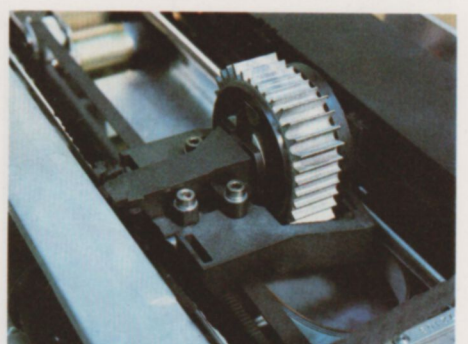
La cabeza de impresión de la PR 1450 consta de nueve agujas que forman matrices de 9 x 7 puntos. Este modelo puede también realizar gráficos por control independiente de las agujas.
