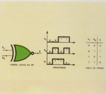
La puerta lógica OR-Exclusiva efectúa la operación de suma lógica exclusiva: el estado lógico de salida será alto cuando las dos entradas reciban estados lógicos distintos.
