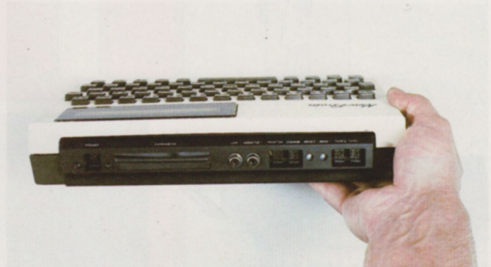
En la zona posterior del mueble que aloja a la unidad central se encuentran los conectores para la comunicación con dispositivos periféricos y memorias de masa.
