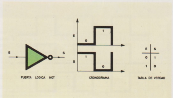
La función lógica de complementación, realizable por una puerta NOT, suele también denominarse negación o inversión. La salida de la puerta NOT entrega el estado lógico opuesto al aplicado en la entrada.
