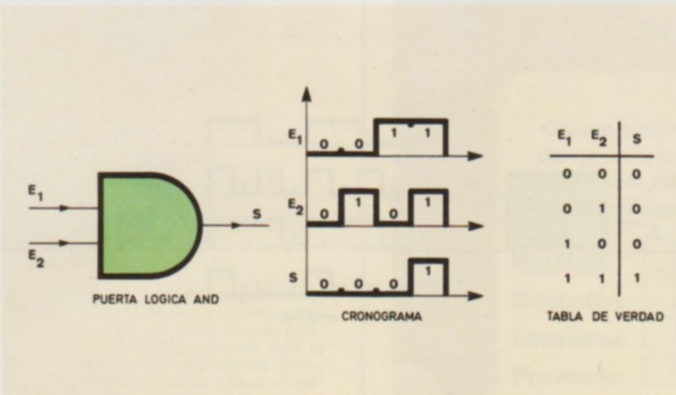
La puerta lógica AND efectúa la operación «producto lógico». La salida estará a nivel lógico alto sólo cuando se aplique un estado alto a ambas entradas.
