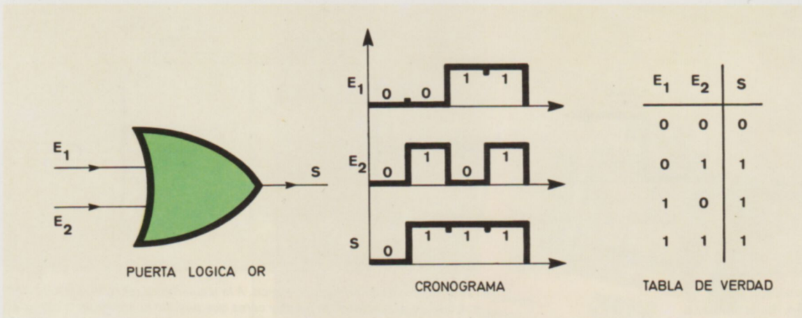
Puerta lógica OR. Realiza la función «suma lógica». La salida del circuito adquiere estado lógico alto, cuando se aplica un estado alto en cualquiera de las dos entradas.
