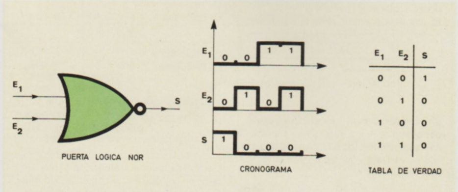
La puerta lógica NOR sintetiza la suma lógica complementada de los estados lógicos aplicados a las líneas de entrada.
