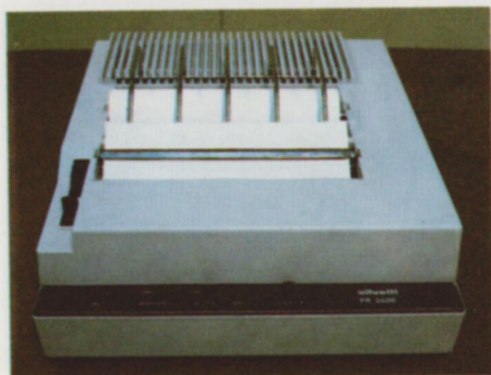
Impresora térmica modelo 2400. Su cabeza consta de 80 electrodos que forman matrices de 7 x 5 puntos e imprimen a razón de 240 líneas, de 80 caracteres, por minuto.
