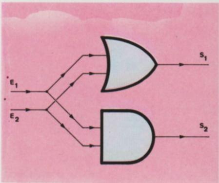
La función lógica f(X_1, X_2) = (X_1 \oplus X_2, X_1 \wedge X_2) puede operarse por medio de un circuito combinacional formado por dos puertas lógicas: La OR, calcula S_1 = X_1 \oplus X_2 , y la AND, S_2 = X_1 \wedge X_2 .
