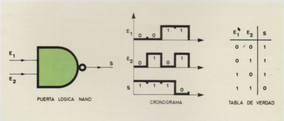
La puerta lógica NAND realiza la operación producto lógico complementado de los estados de entrada.
