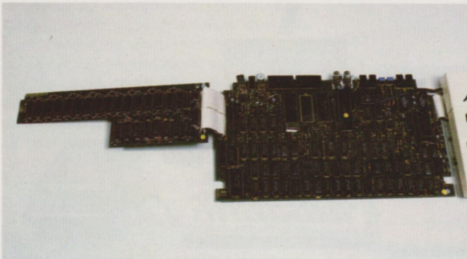
La unidad central del New Brain está basada en el popular microprocesador de 8 bits Z-80 A de la firma Zilog. La máxima zona de memoria RAM direccionable por el equipo es de 2 Mbytes.
