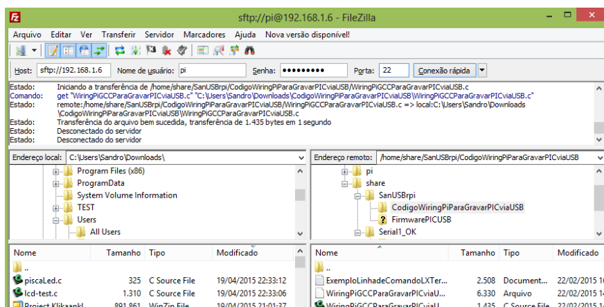
Figura 18.1: Filezilla.
