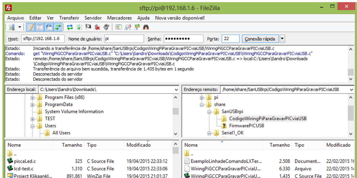
Figura 5.13: Filezilla
