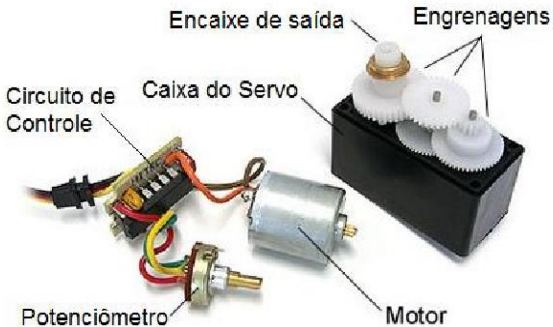
Figura 12.2: Servo Motor
