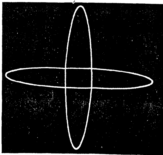
3.111 Oszillografische Abstimmmanzeige beim Filterkonverter: Exakte Abstimmung, da die Ellipsen senkrecht aufeinander stehen. Ellipsenbildung durch Übersprechen der beiden Kanäle.
