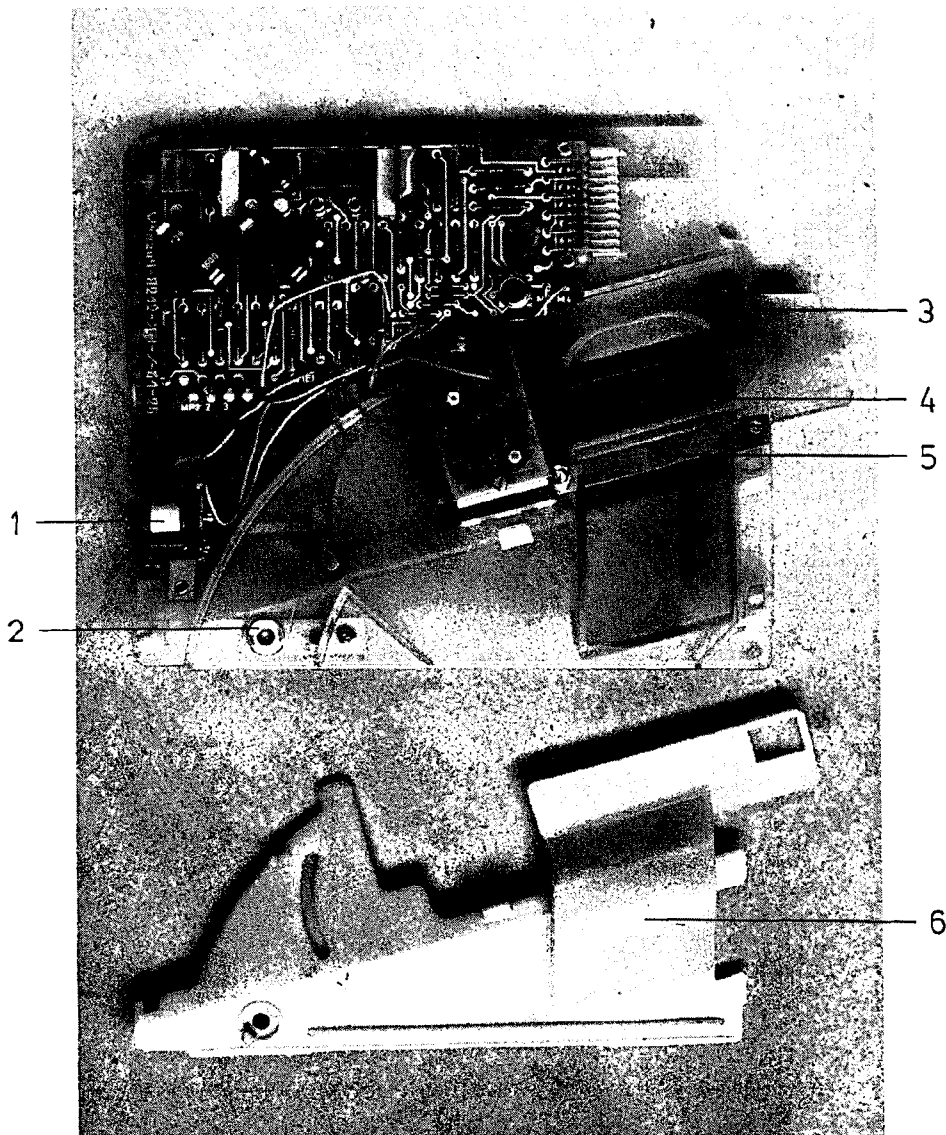
Bild 9: Münzprüfer (Baugruppen 2, 3, 4)
