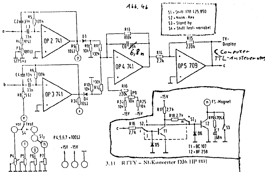
3.11 RTTY-NF-Konverter DJ6 HP 001 Abb. 4 a
