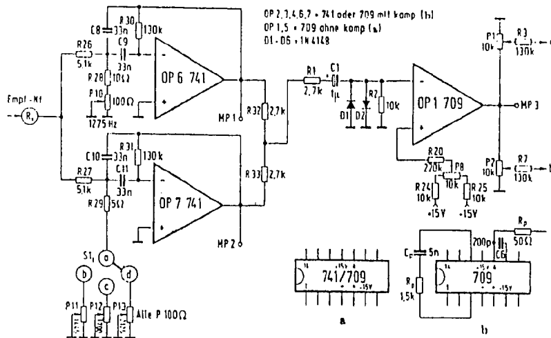
3.11 RTTY-NF-Konverter DJ6 HP 001 Abb. 4 a
