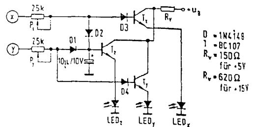
3.116 LED-Abstimmmanzeige für Filterkonverter
