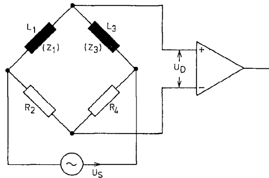
Bild 10: Grundsätzlicher Aufbau der Münzprüferbrücke
