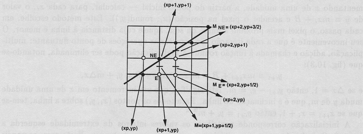
Figura 10.4: Algoritmo do Ponto Médio.
