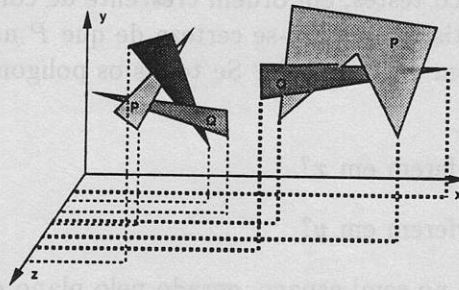
Figura 11.5: Casos em que um Ciclo Infinito Ocorre se não Houver Marcação.
