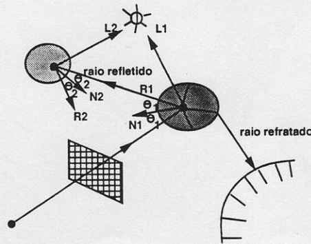
Figura 13.3: Traçado de Raios.
