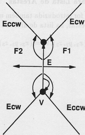
Figura 6.4: Codificação por Arestas Aladas.
