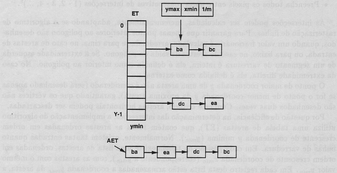
Figura 10.9: Tabela de Arestas e Tabela de Arestas Ativas.
