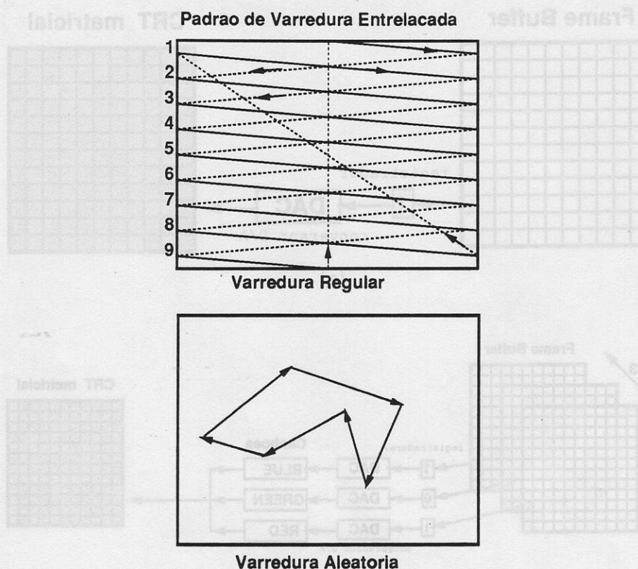
Figura 3.8: Padrões de Varredura.
