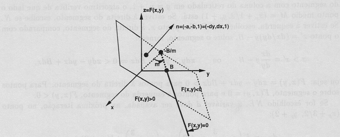
Figura 10.5: Gráfico da função F(x, y) .
