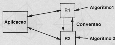
Figura 6.7: Multi-representação.
