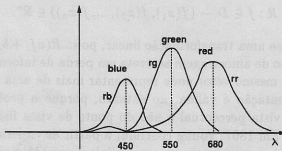
Figura 2.5: Funções de Reconstrução de Cor.
