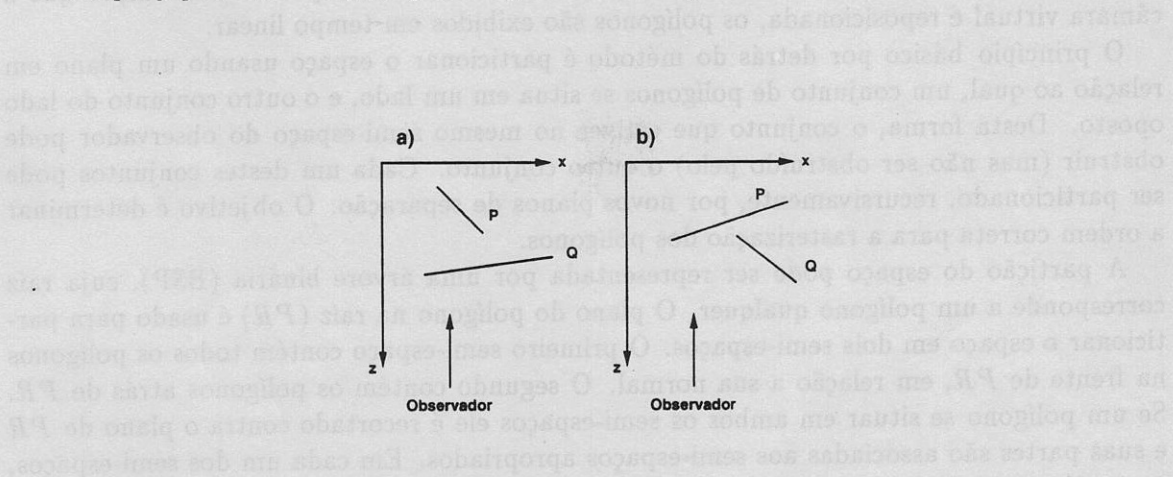
Figura 11.4: Teste 3 e 4.
