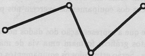
Figura 3.2: Formato Vetorial.
