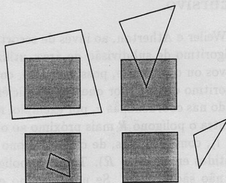
Figura 11.6: Quatro Relações de Polígonos com um Elemento de Área.
