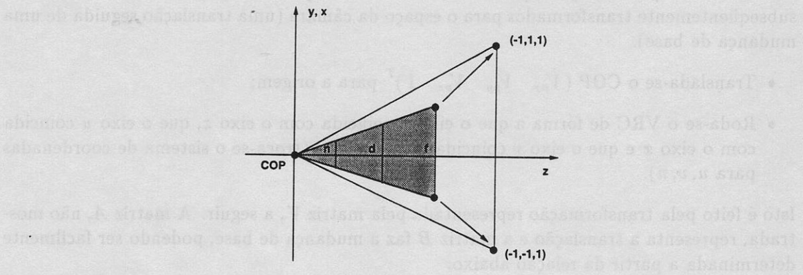
Figura 8.4: Escala.
