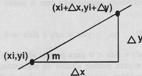
Figura 10.3: Coeficiente Angular de um Segmento.
