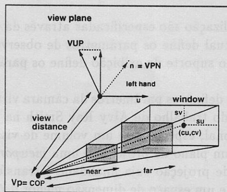
Figura 8.2: Sistema de Coordenadas da Câmara.
