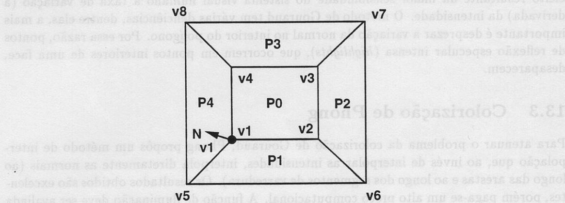
Figura 13.2: Cálculo da Normal em um Vértice.
