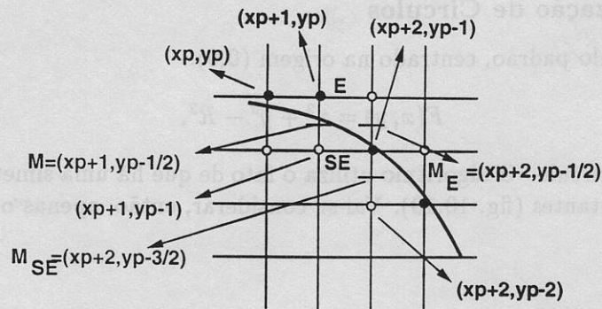
Figura 10.11: Algoritmo do Ponto Médio para Círculos.
