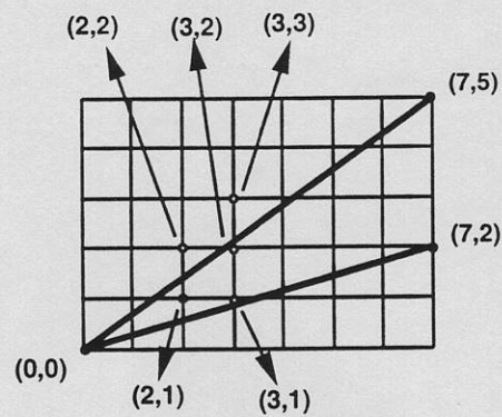
Figura 10.17: Casos Degenerados no Algoritmo do Ponto Médio para Retas.
