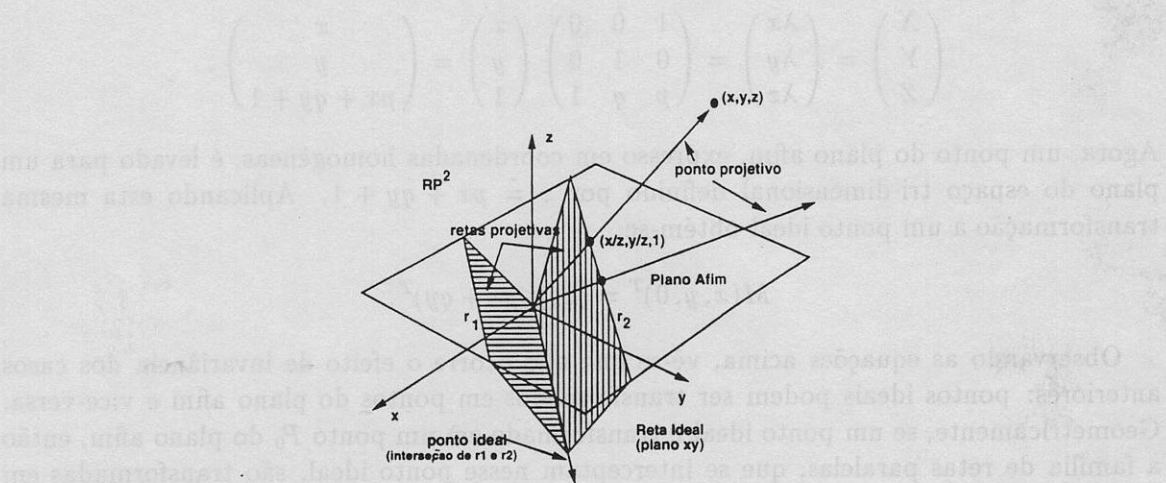
Figura 5.4: Plano Projetivo.
