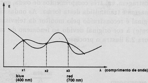
Figura 2.4: Representação Finita de duas Funções.
