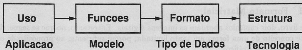
Figura 3.1: Modelo Conceitual.
