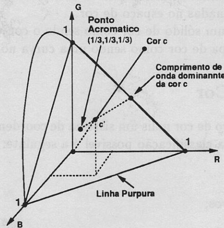
Figura 2.8: Diagrama de Cromaticidade.
