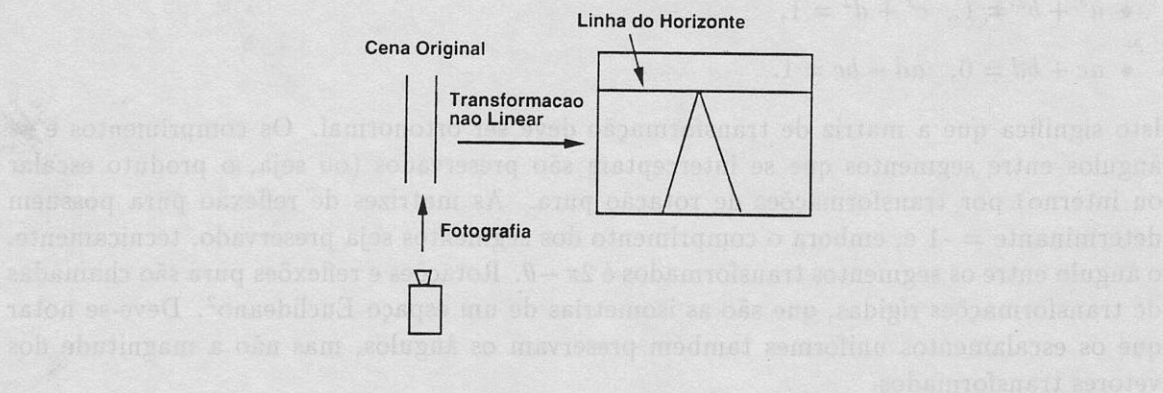
Figura 5.3: Transformação Projetiva.
