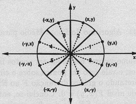
Figura 10.10: Simetria em um Círculo.
