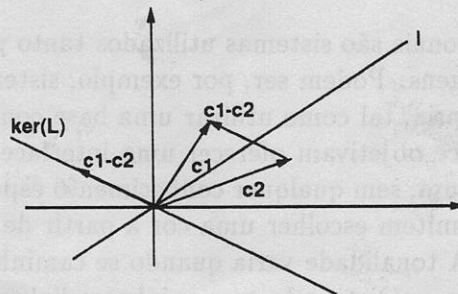
Figura 2.9: Decomposição Crominância-Luminância.
