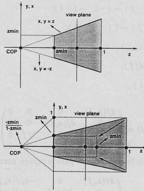
Figura 8.5: Transformação Perspectiva.
