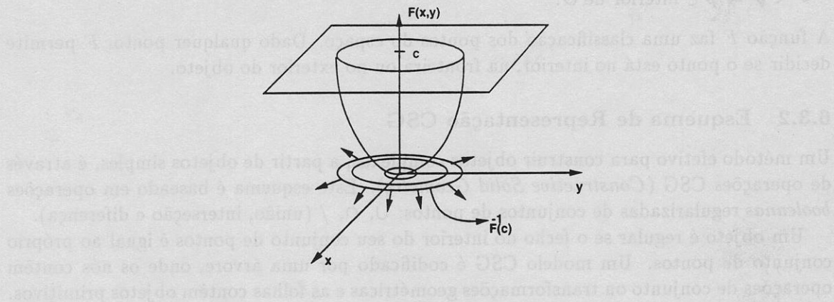
Figura 6.5: Círculo Definido Implicitamente.
