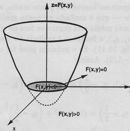
Figura 10.12: Gráfico da Função F(x, y) .
