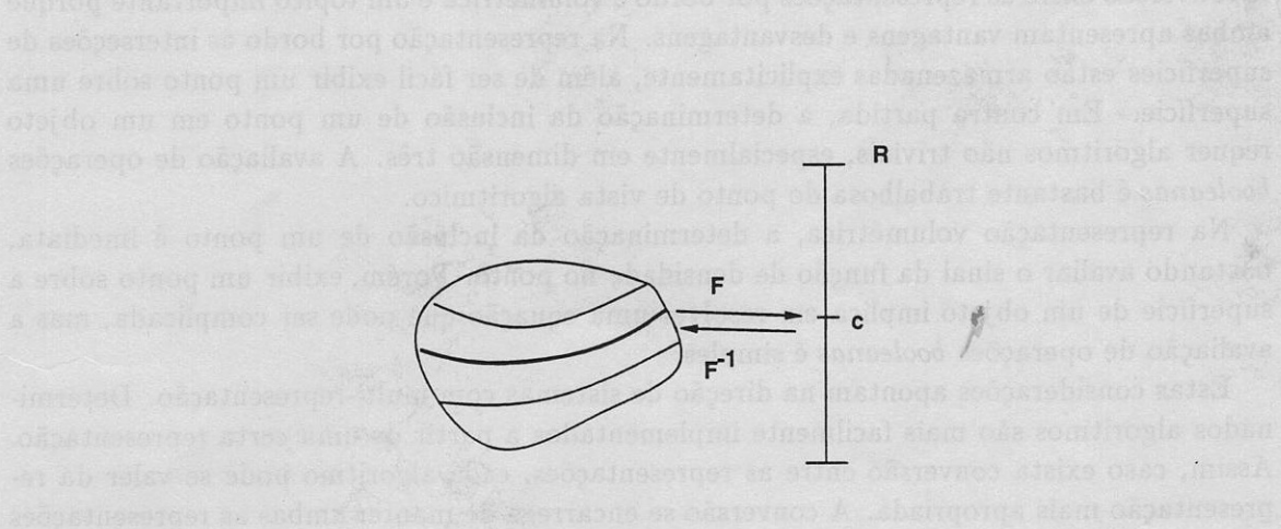
Figura 6.6: Objeto Implícito.
