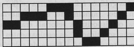
Figura 3.3: Formato Matricial.
