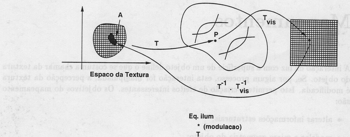
Figura 14.1: Mapeamento.
