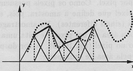
Figura 10.14: Interpolação Linear.
