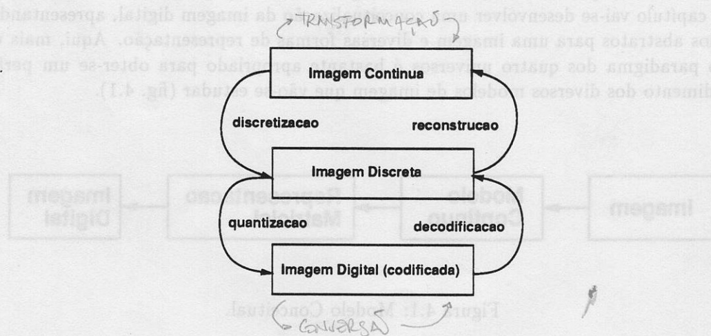
Figura 4.2: Imagem Digital.
