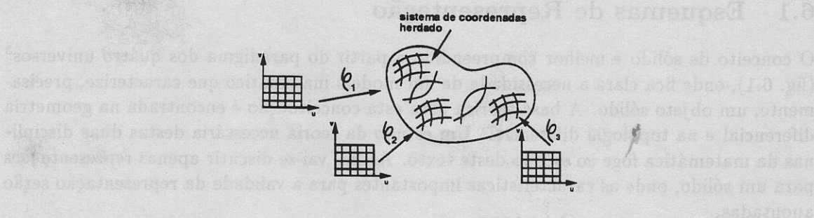
Figura 6.2: Parametrização de uma Superfície.
