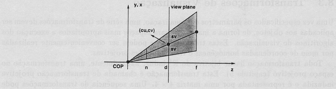
Figura 8.3: Cizalhamento.
