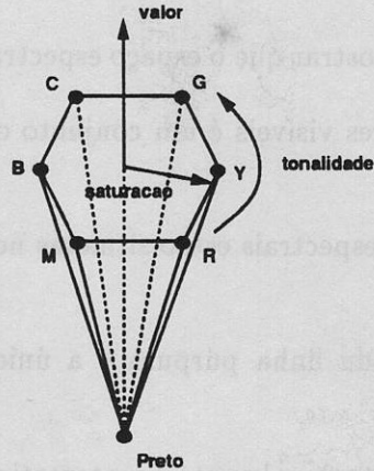
Figura 2.10: Sistema HSV.
