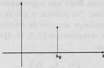
Figura 2.6: Cor Espectral.
