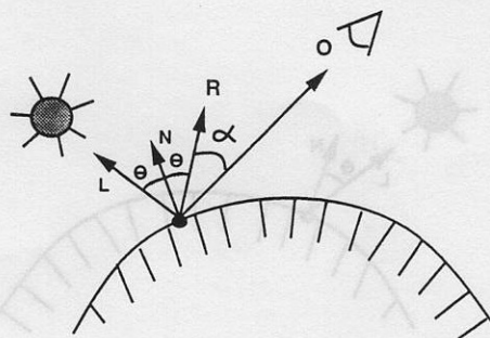
Figura 12.5: Modelo de Phong.
